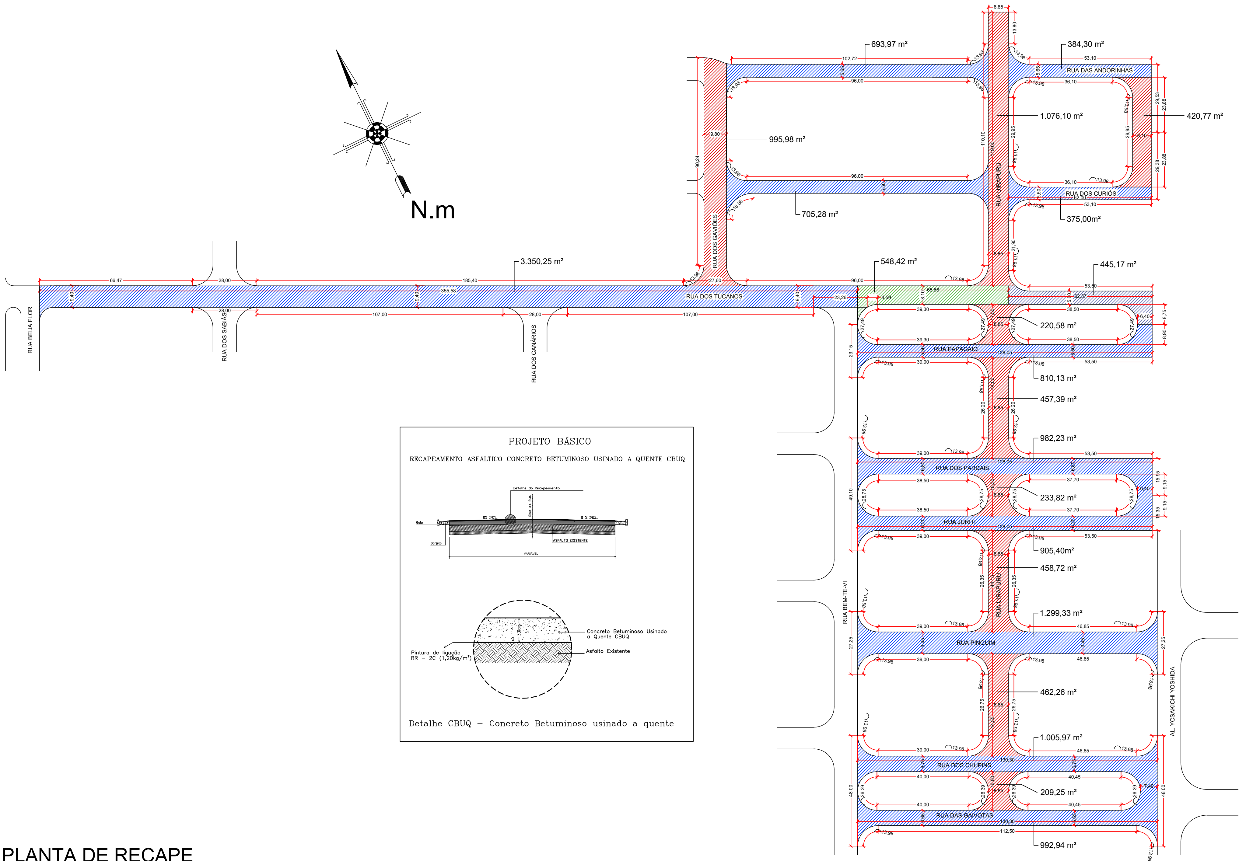
PLANTA DE RECAPE ESC.: 1/1000
