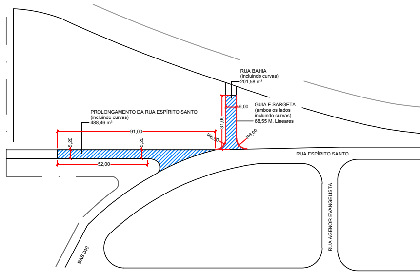
PLANTA DE PAVIMENTAÇÃO ESC.: 1/1000
