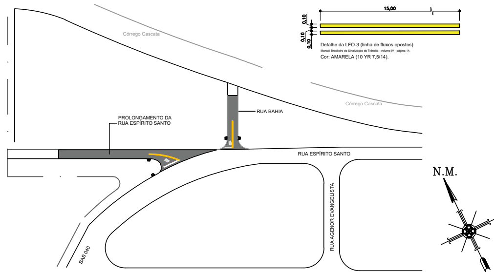
SINALIZAÇÃO HORIZONTAL ESC.: 1/1000
