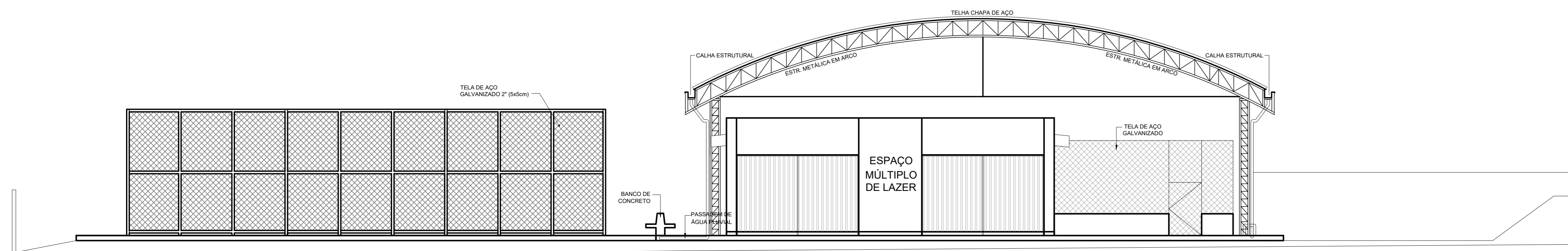
FACHADA RUA DAS CAMÉLIAS escala: 1/75
