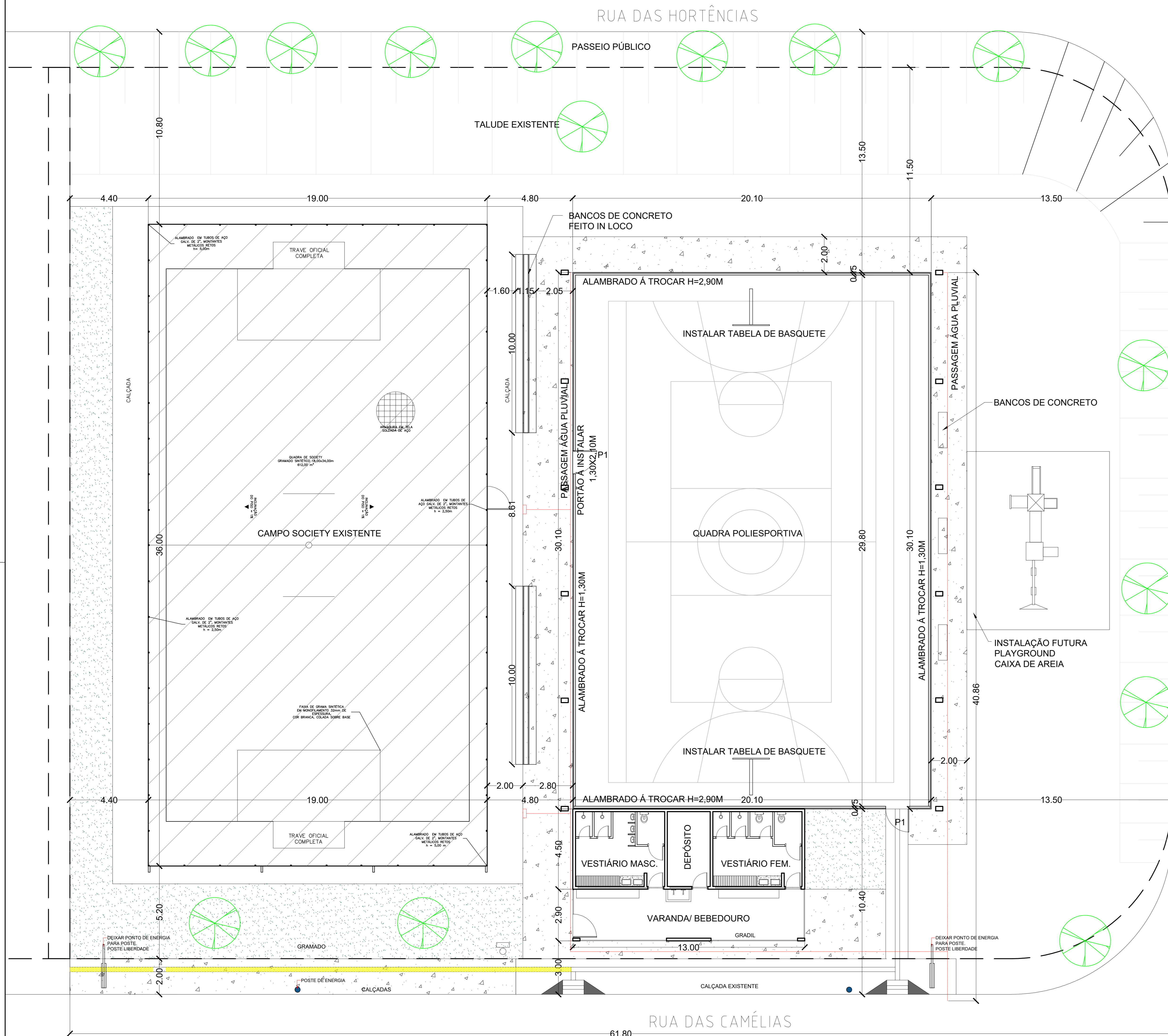
PLANTA escala: 1/100
