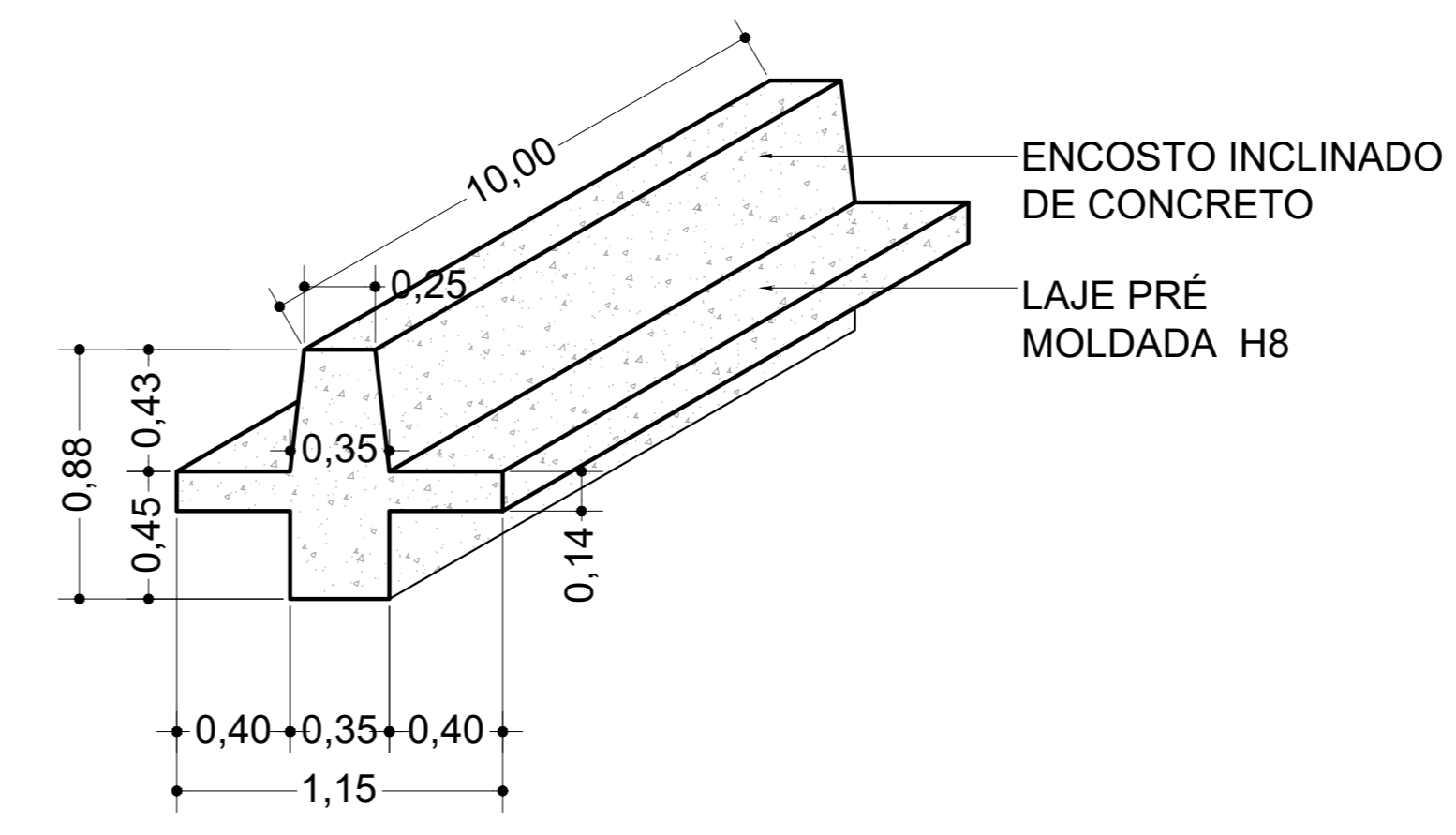
ISOMÉTRICA BANCO escala: 1/25
