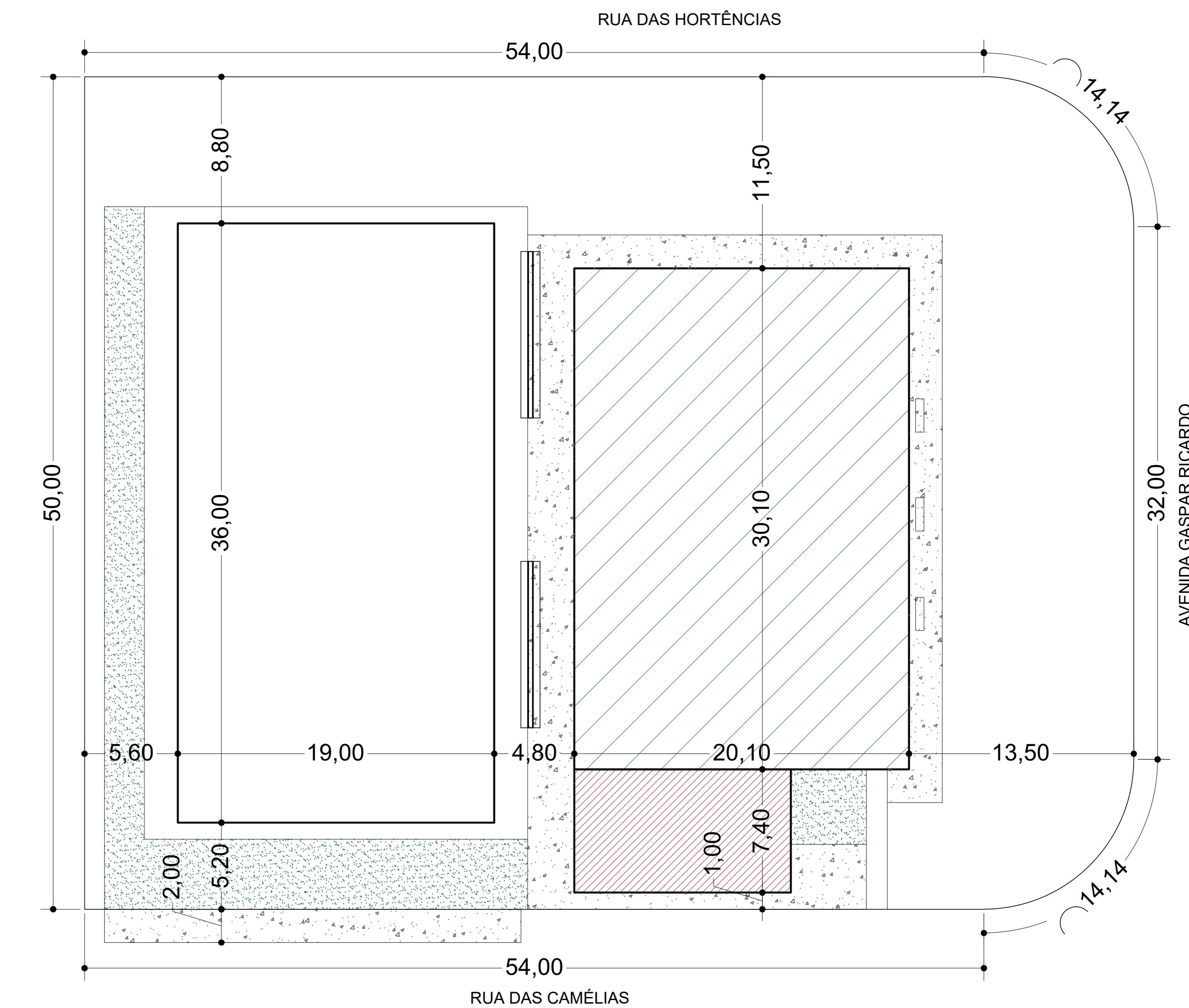
IMPLANTAÇÃO escala: 1/200
