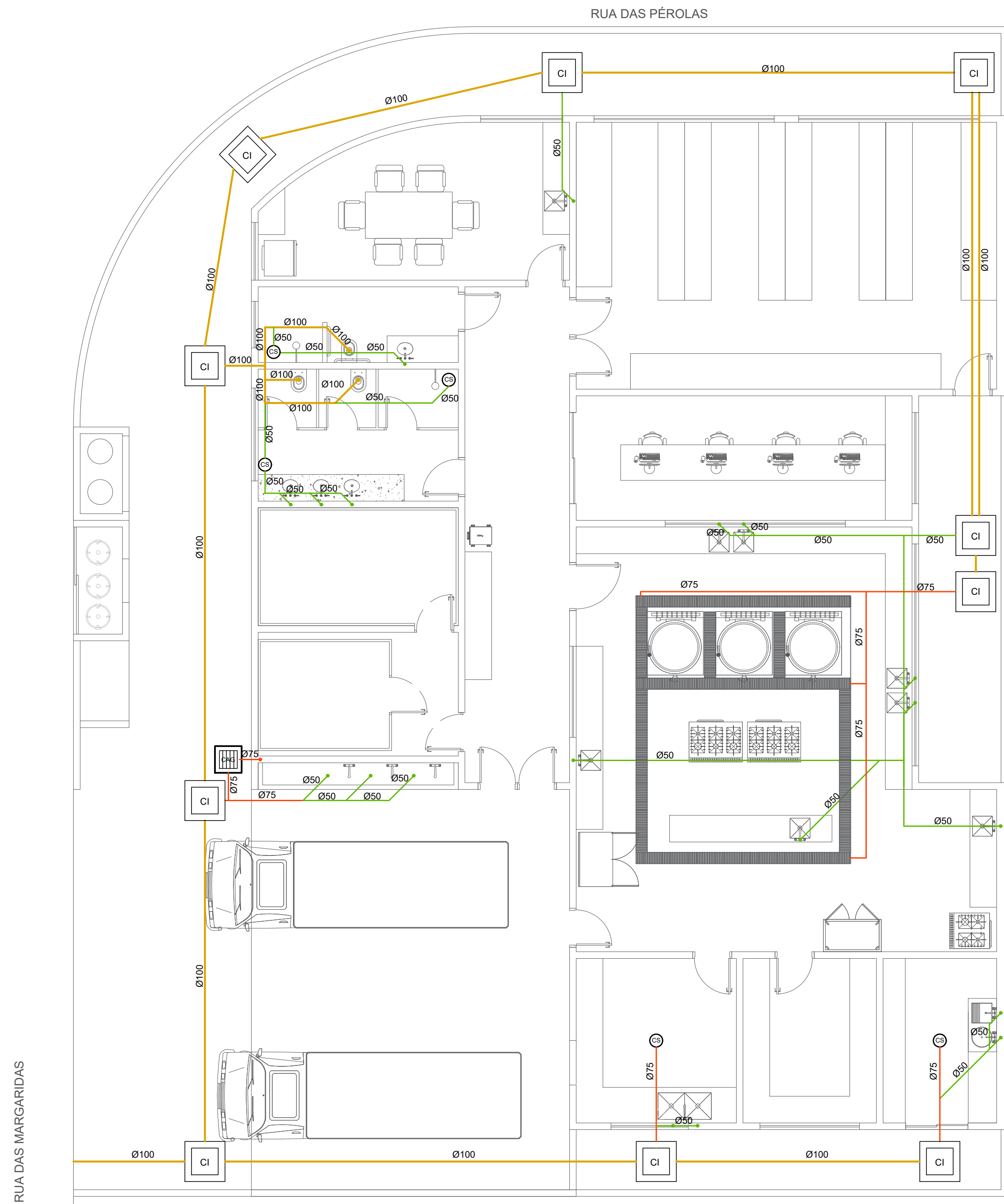
PLANTA REDE DE ESGOTO escala: 1/75
