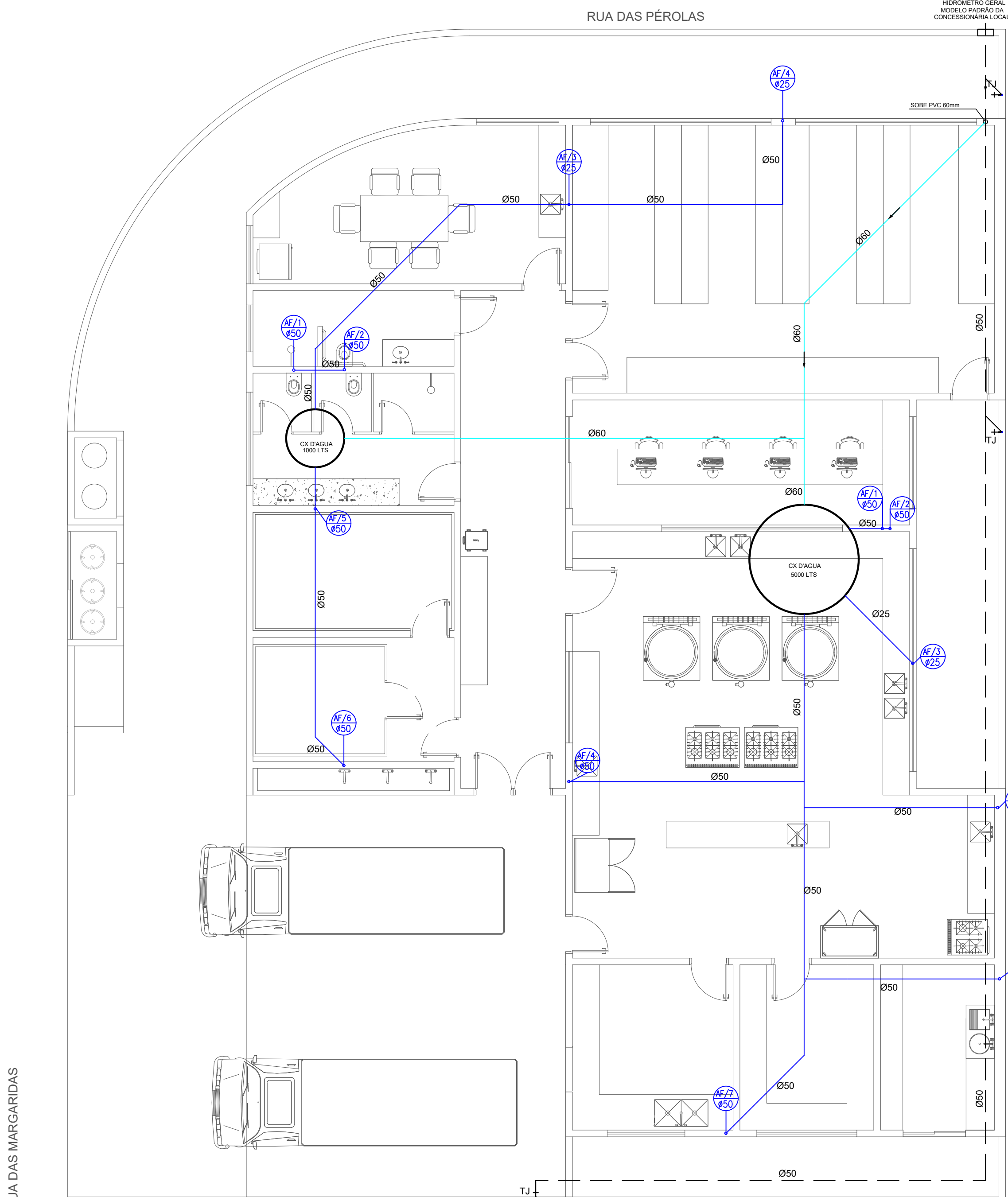
PLANTA REDE DE ÁGUA escala: 1/75
